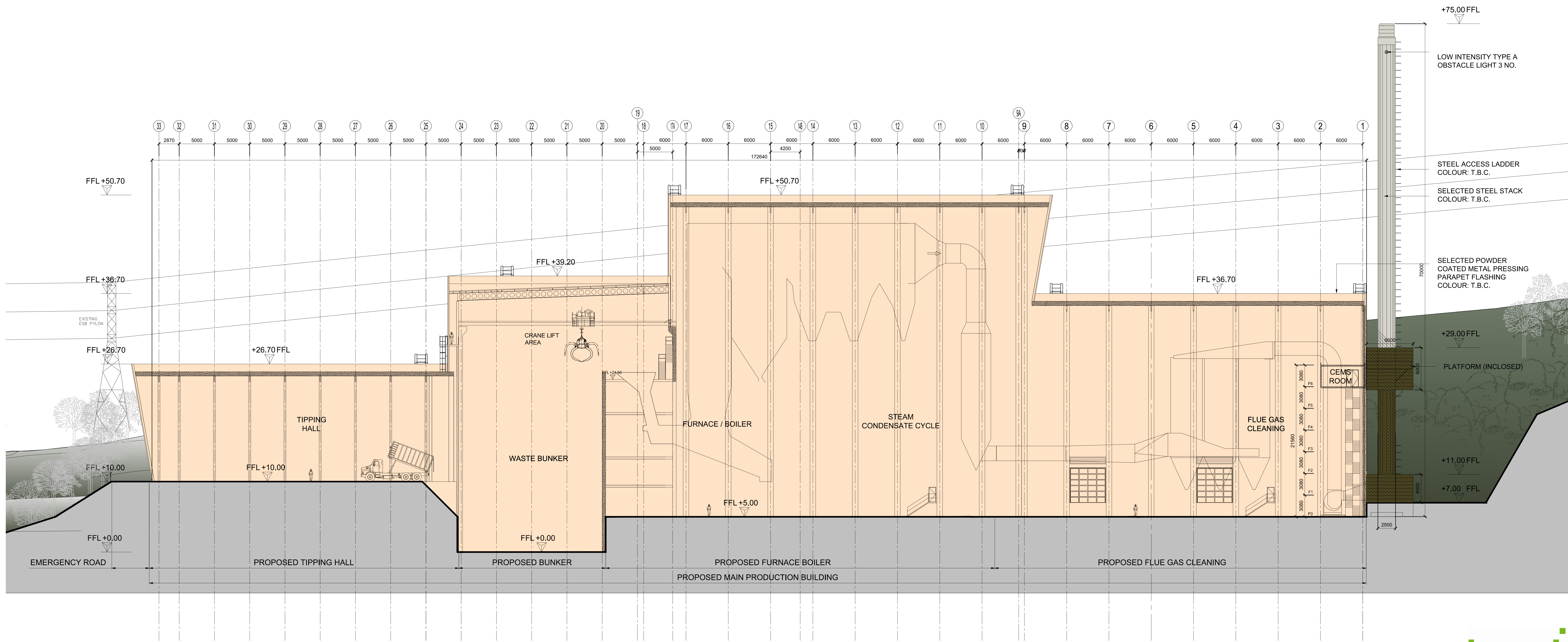
SECTION CC (SCALE 1:200 @A0)
